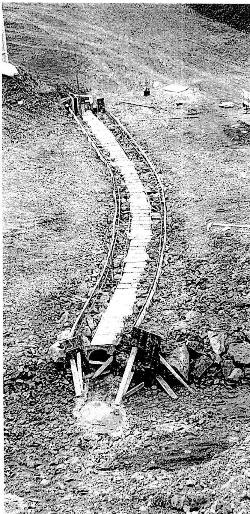
EXECUÇÃO DE TUBULAÇÃO NA GRANJA FARADAY NÚCLEO 1 - CAPANEMA
